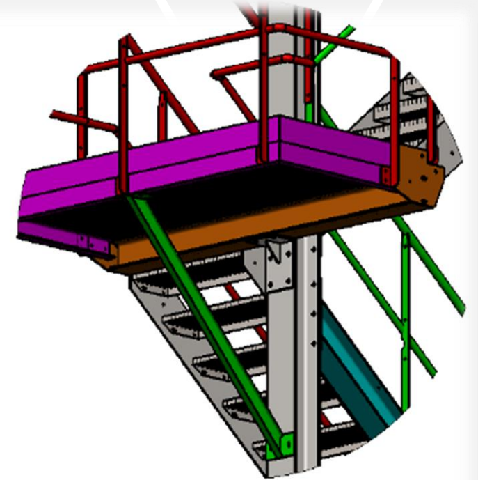
DÉTAIL H PLATEFORME 2
